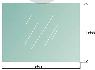
Glass tolerances EN 572-2
